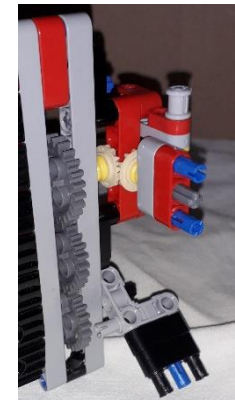
Prevodovka
